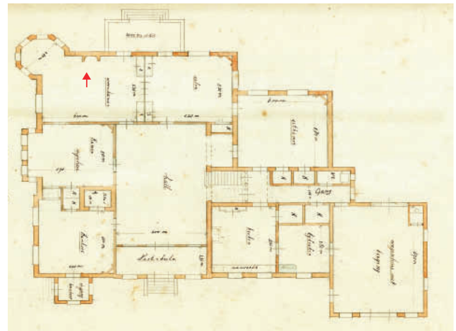
5a Woning en kantoor voor notaris mr C. de Ranitz, Hoofdstraat West 70, Winsum, 1911, noordgevel en begane grondplan (thans gemeentehuis, afbeelding 113).
